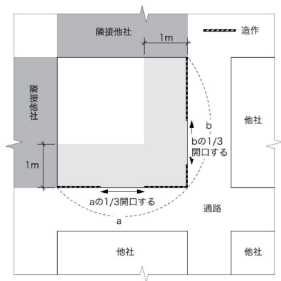
<平面図例>
