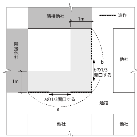
〈平面図例〉
