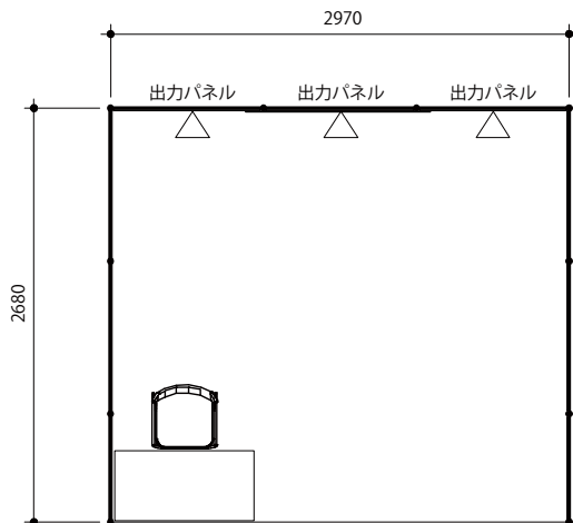
【平面図】
